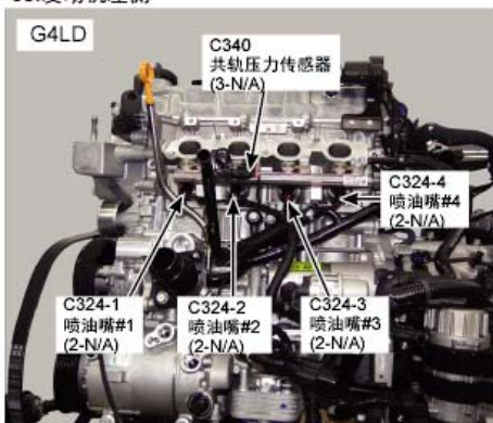
65. 发动机左侧
