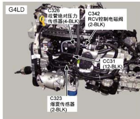
63. 发动机左侧
