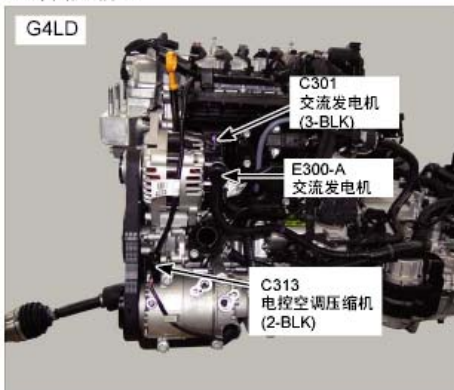
62. 发动机前左
