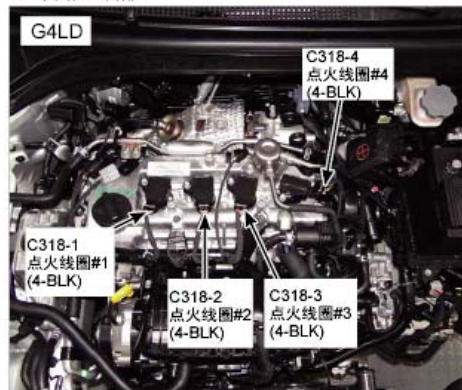
61. 发动机顶部
