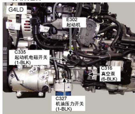
64. 发动机左侧
